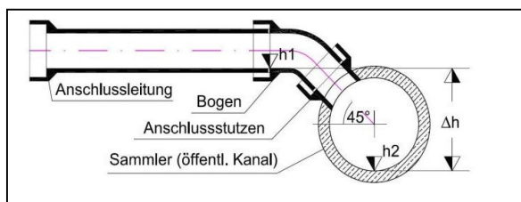
Detailzeichnung (M 1:25)
