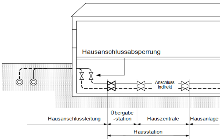
Abb. 1: Hausanschlussleitung und Hausstation nach AGFW FW 515
